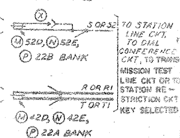
FIG. 2 BANK MULTIPLE NO. 711A, 701B, 711A, 711B OR 710E
