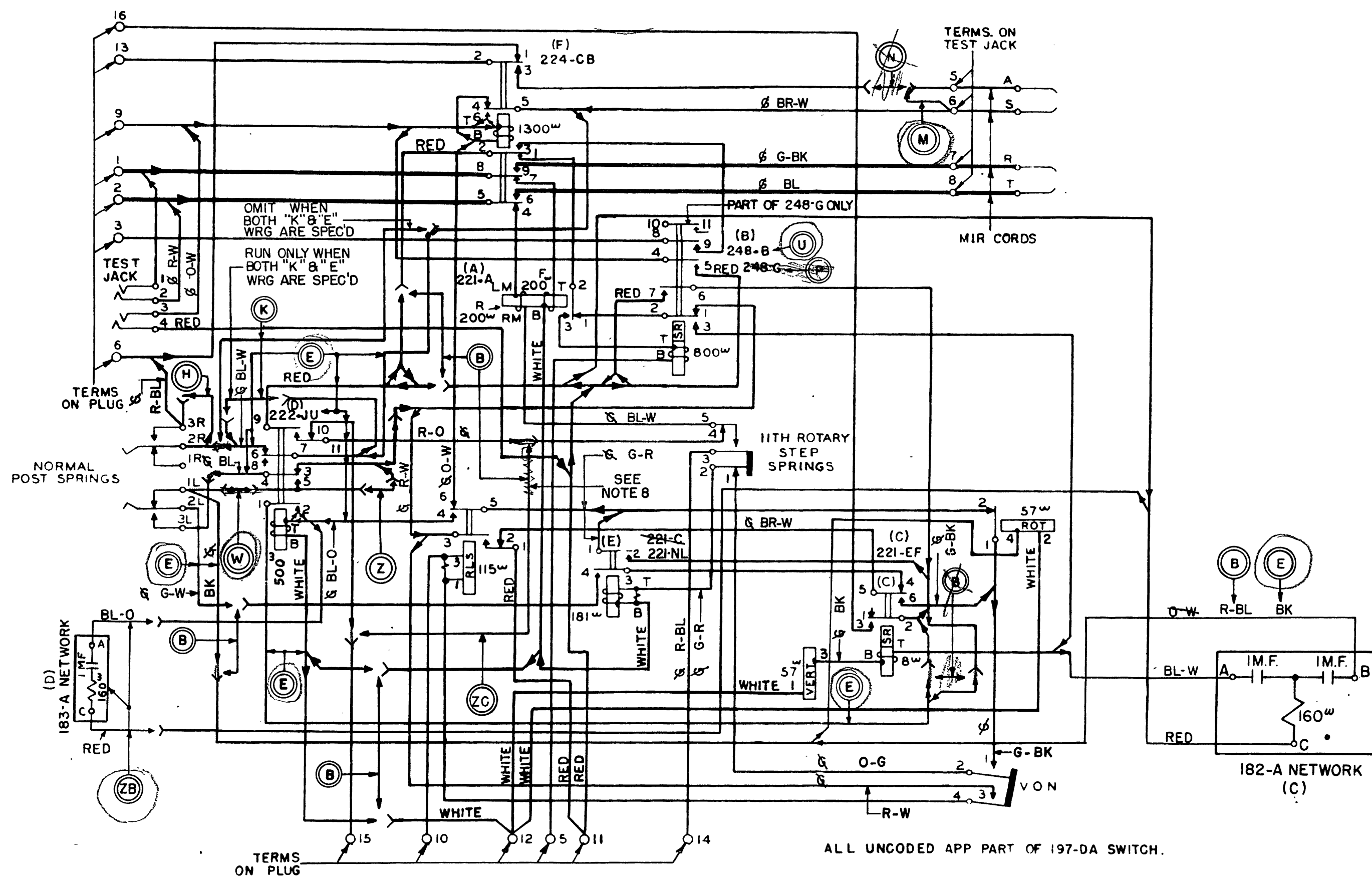
SELECTOR CKT.
